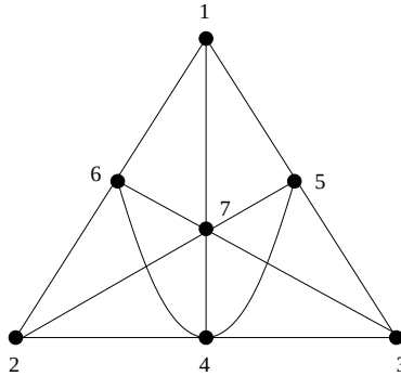
FIGURE 13 – Représentation euclidienne de F_7 .
